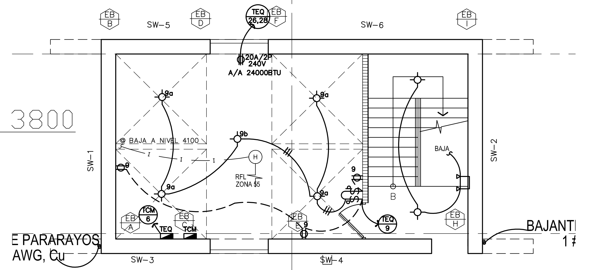
PLANTA DE ELECTRICIDAD NIVEL 3100 @ 3800
