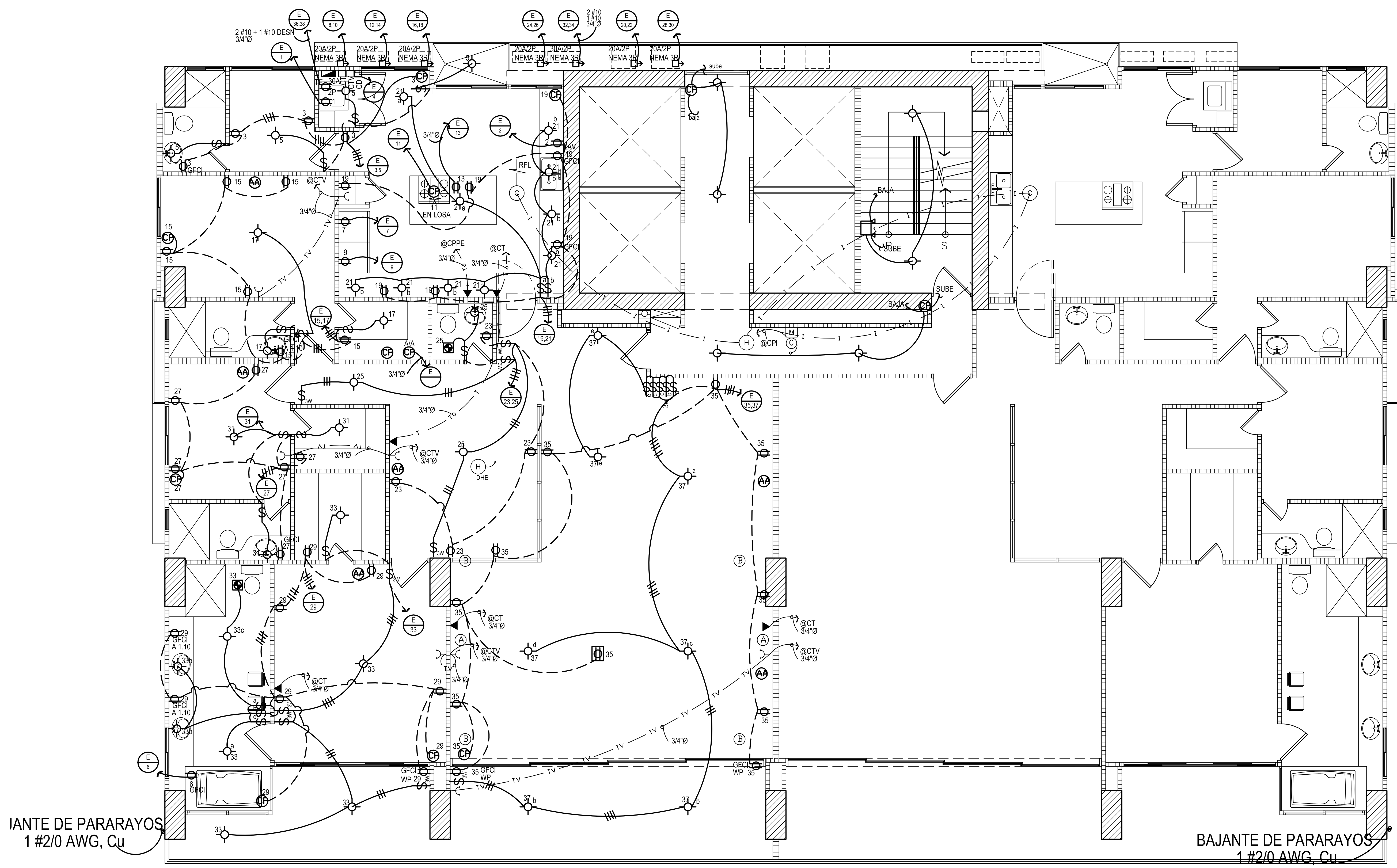
PLANTA DE ELECTRICIDAD NIVEL 3100 @ 3800
