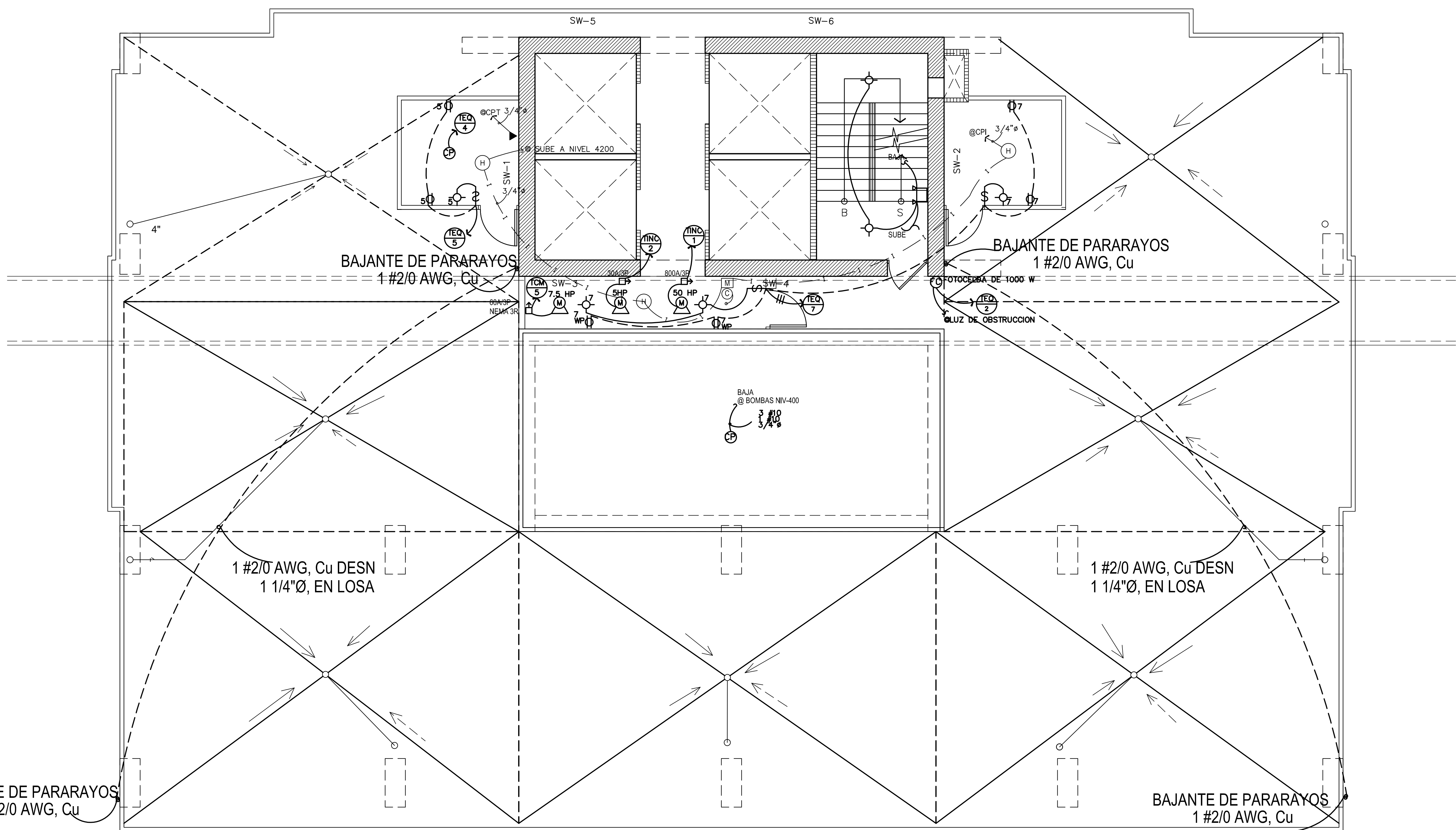
PLANTA DE ELECTRICIDAD NIVEL 3900
