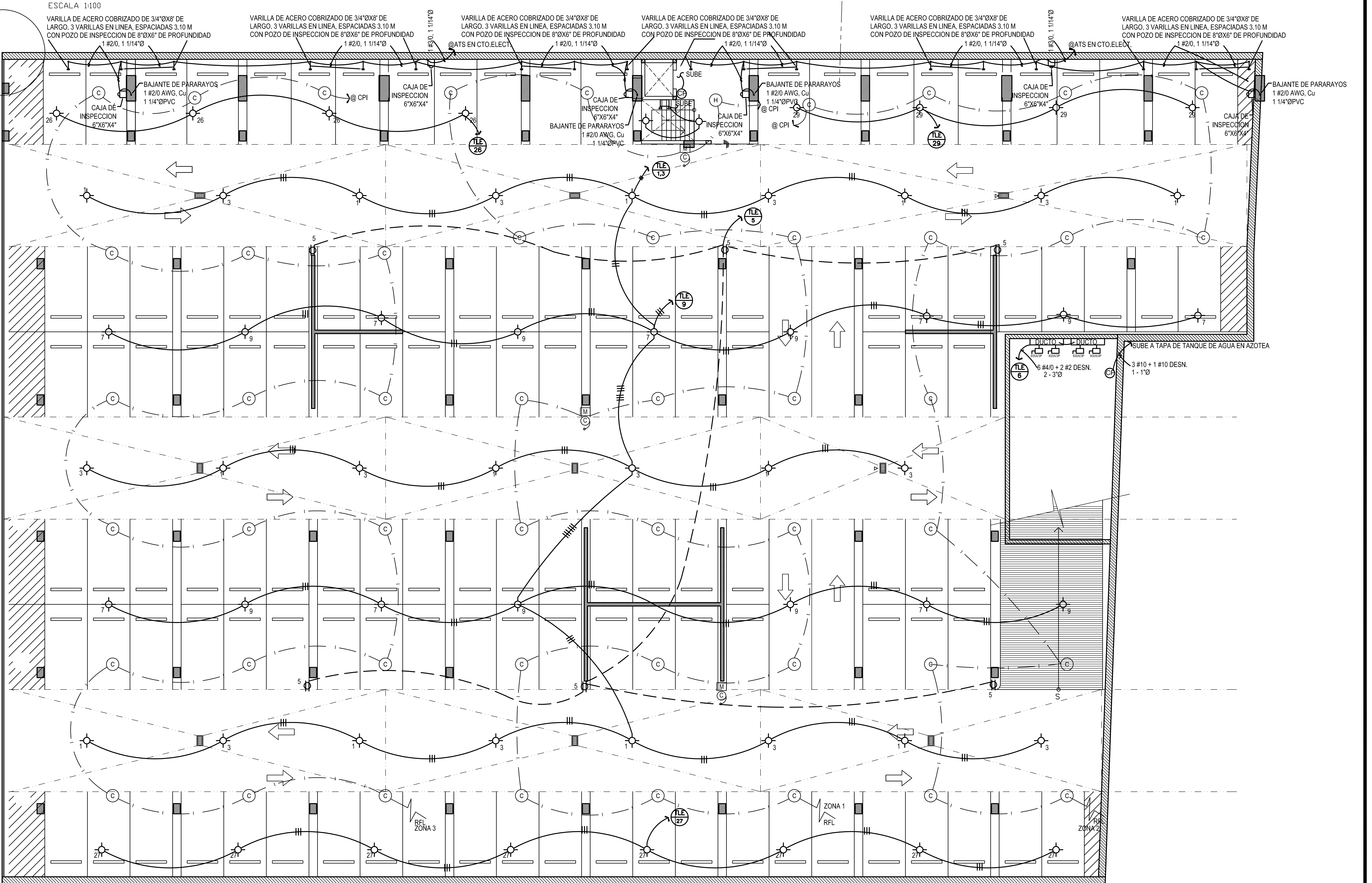
PLANTA DE SOTANO- 400
