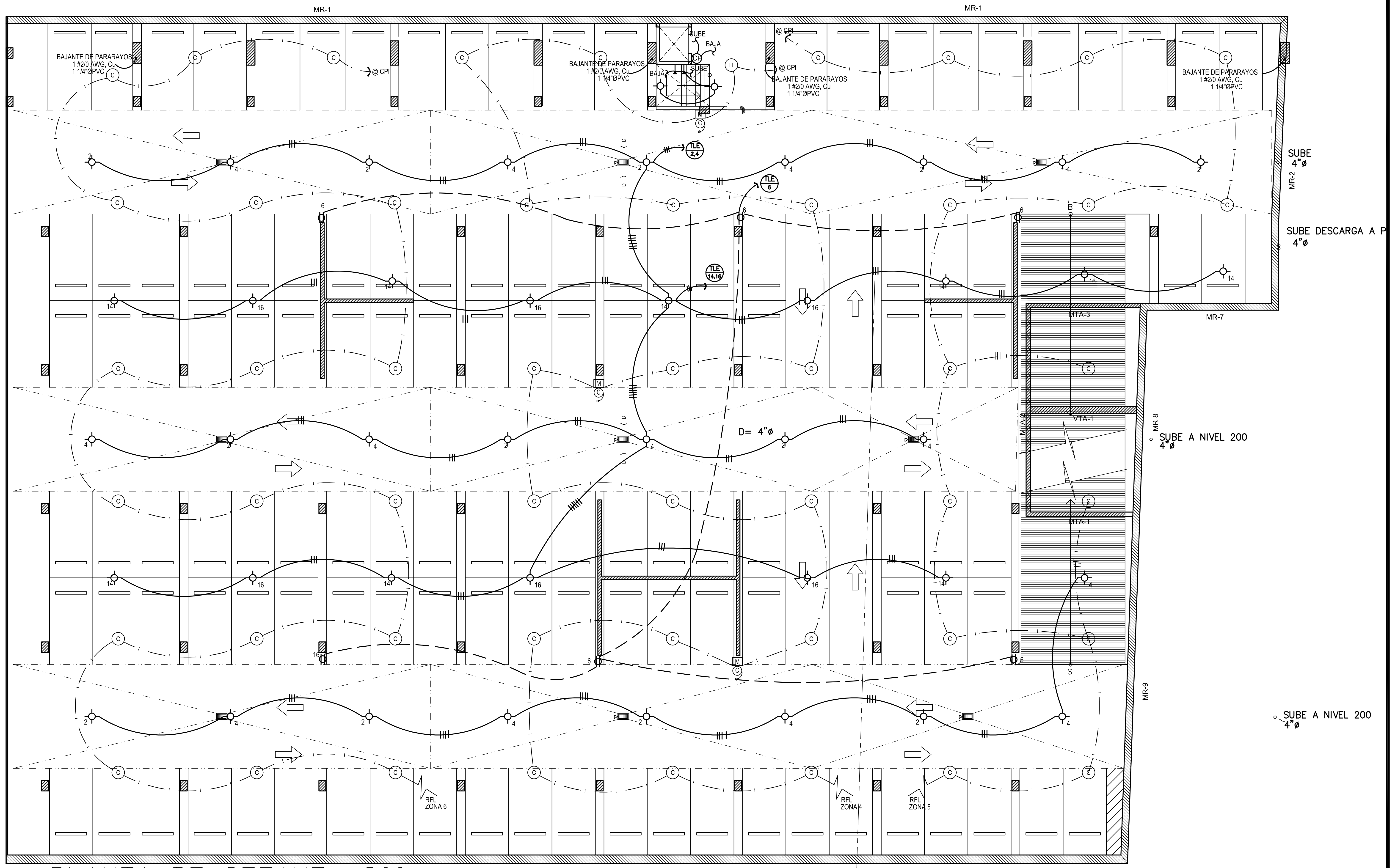
PLANTA DE SOTANO- 300
