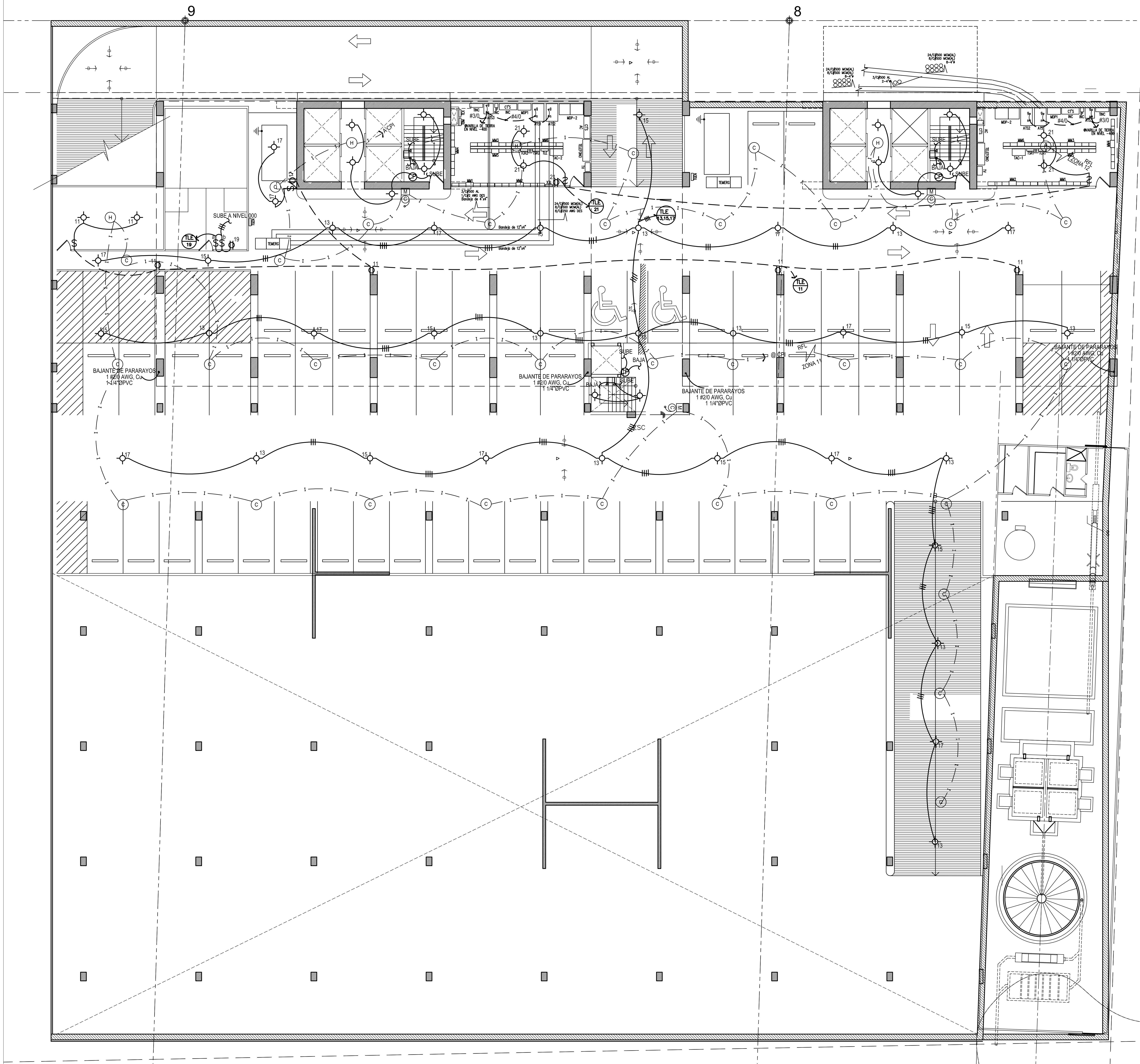
PLANTA DE SOTANO- 100 ESCALA 1:100
