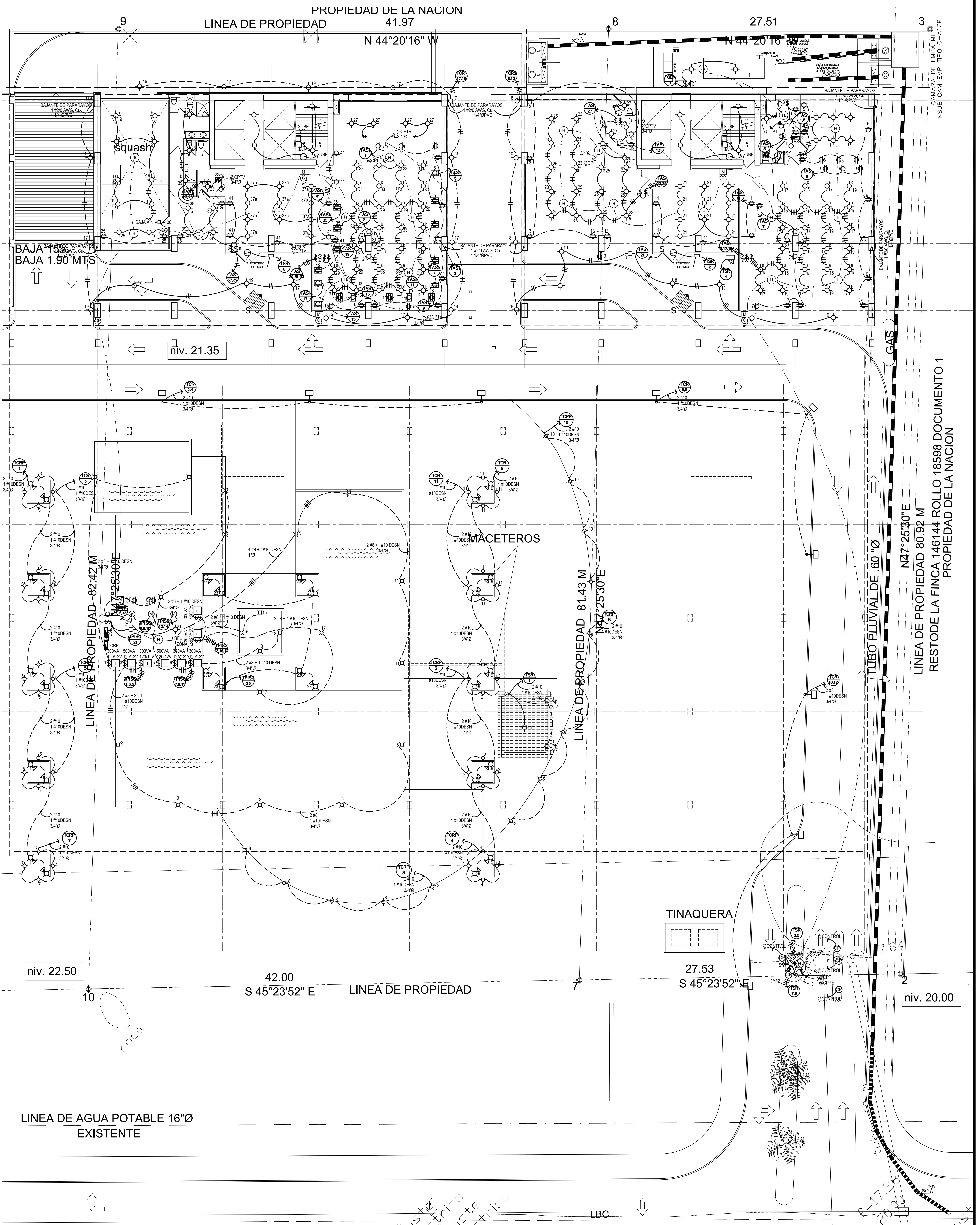
PLANTA DE LOCALIZACION ESCALA 1:100
